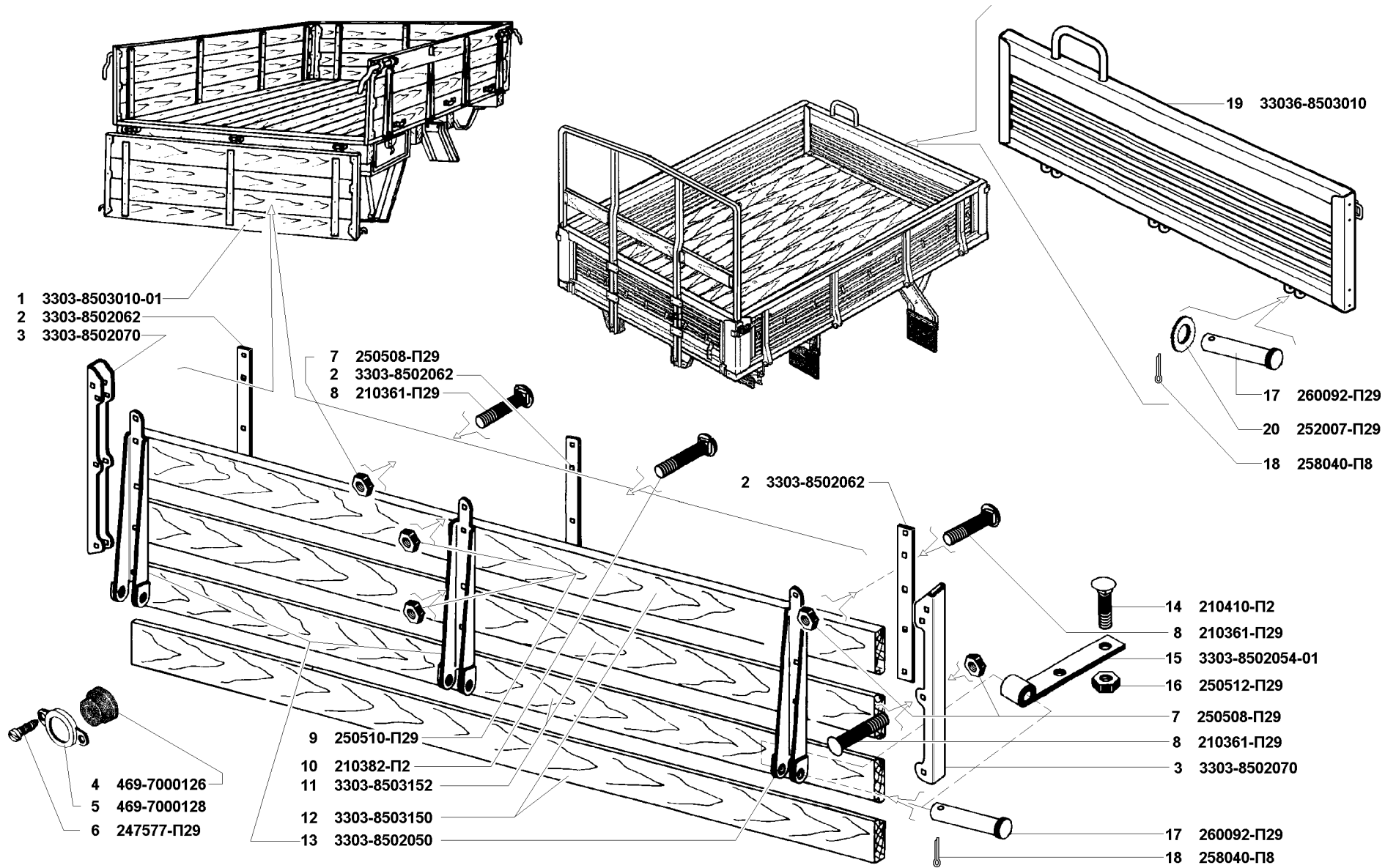
Рис. 159. Борд платформы задний (8503) Fig. 159. Platform tailgate (8503)
